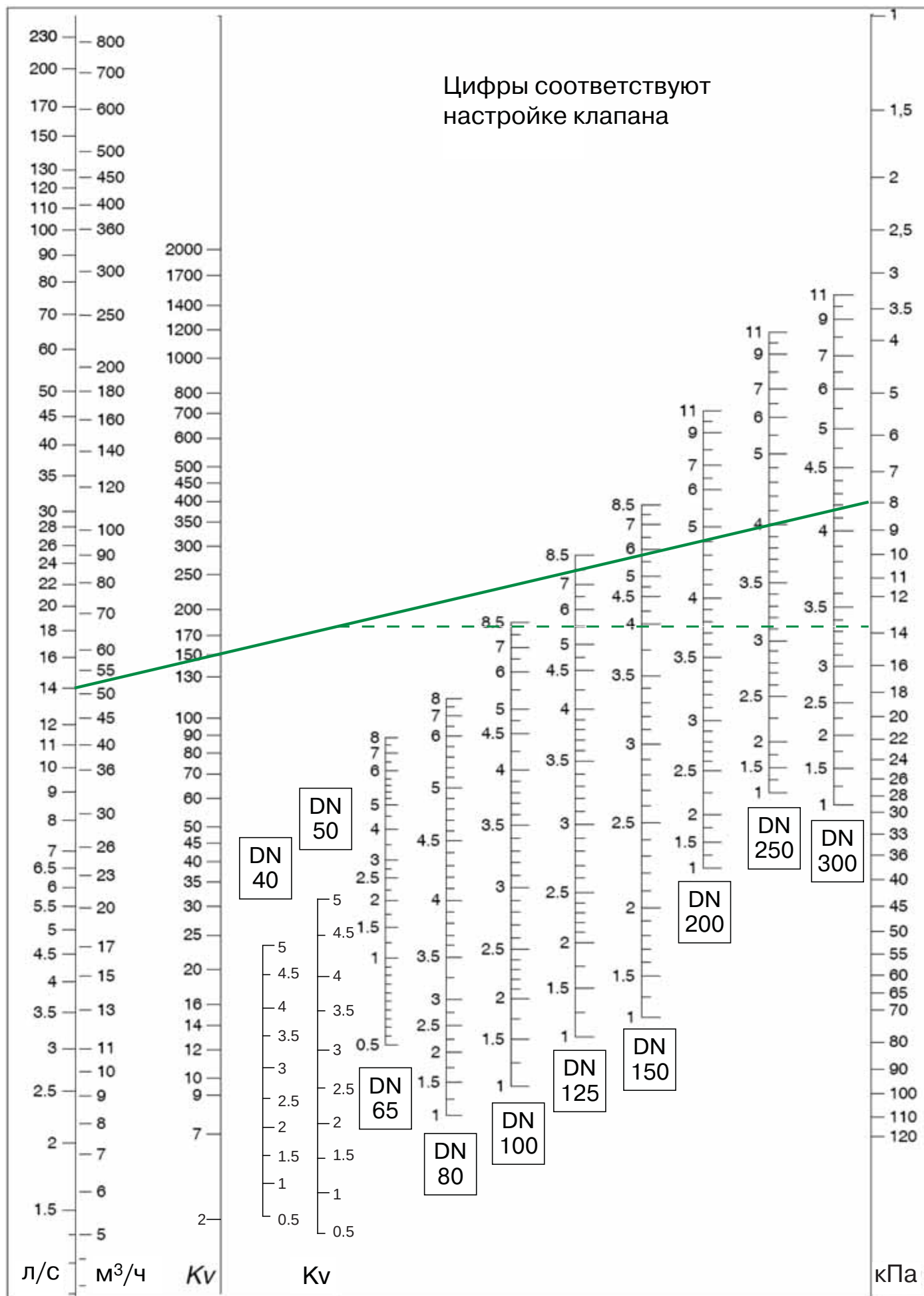
Диаграмма 4. Подбор типоразмера и предварительной настройки клапана
