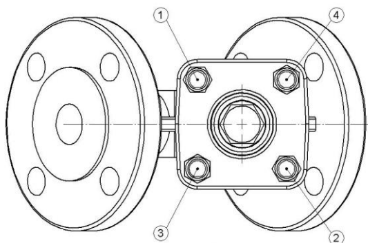
Моменты закручивания болтов
