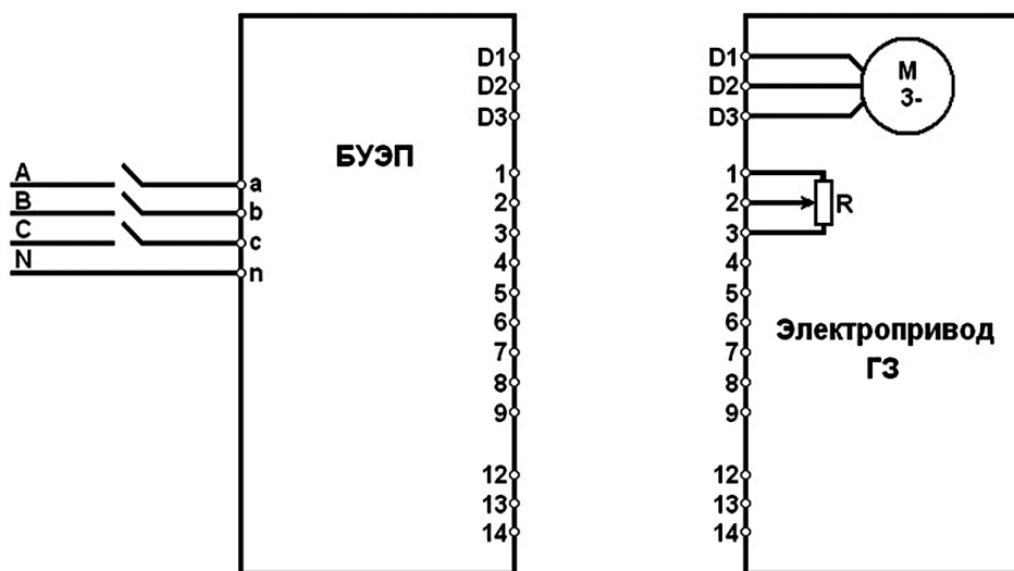
Рис.5 (1) Блок-схема подключения БУЭП к электроприводу (для электросхемы на рис.4 (1))
