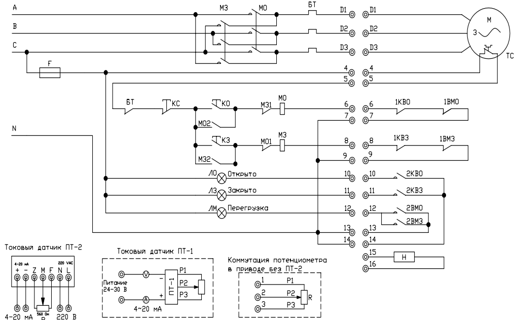
Рис.4 (2) Электрическая схема управления (обновленная схема)
