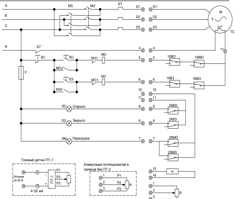
Рис.4 (1) Электрическая схема управления
